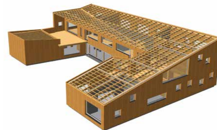
3D-VISUALISIERUNG: SÜD-OST-ANSICHT
