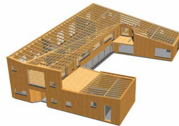
3D-VISUALISIERUNG: SÜD-WEST-ANSICHT
