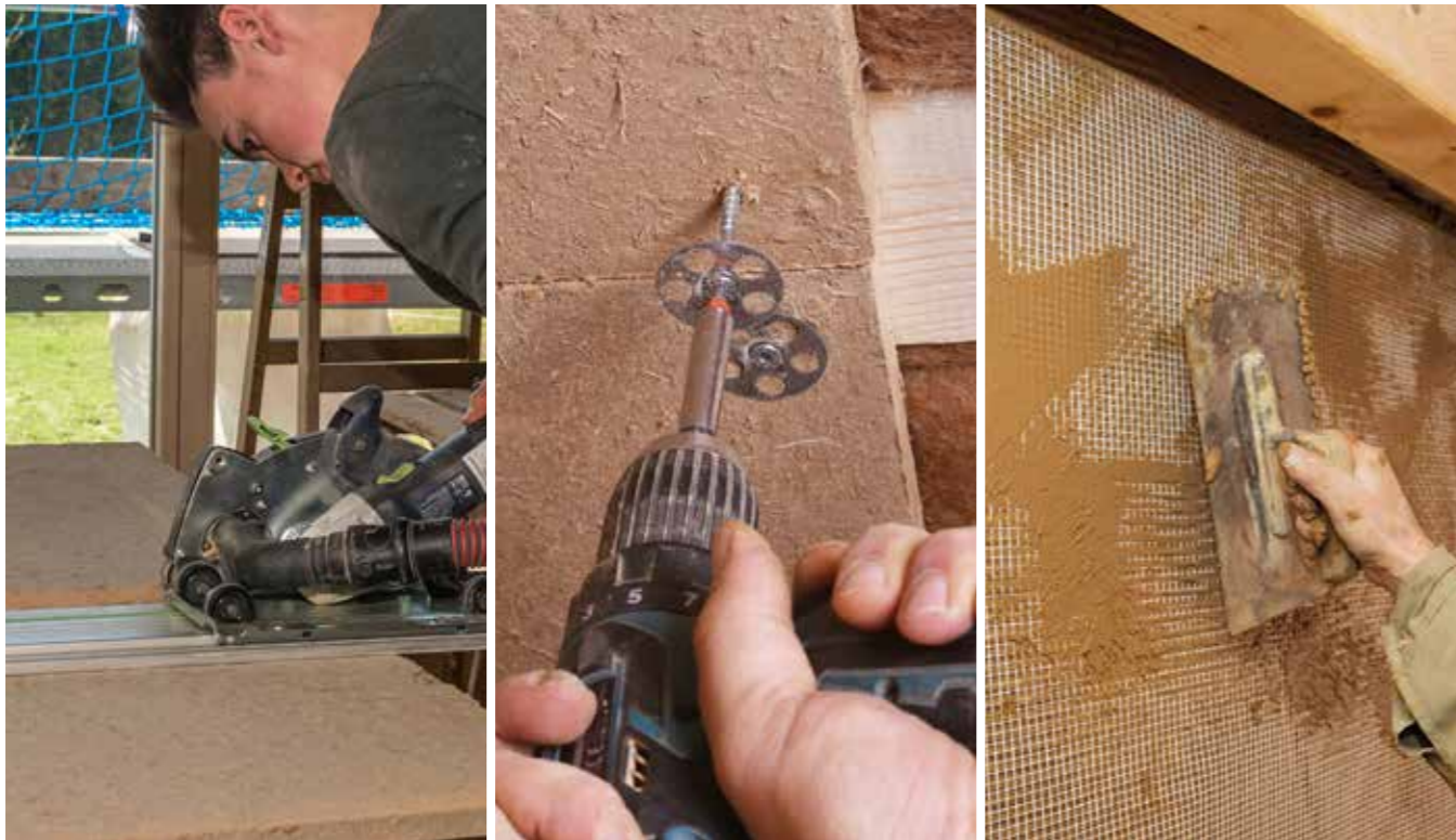
BU: Der passgenaue Zuschnitt der Agaton Lehmplatten erfolgt mit üblichen Werkzeugen wie beispielsweise einer Kreissäge. Die Lehmplatten können zur Befestigung geklebt, geklammert oder geschraubt werden. Final werden die Lehmplatten mit einer nur fünf bis acht Millimeter starken Oberputzschicht versehen. Als vollflächige Armierung dient Glasseidengewebe. Bilder: tdx/Thermo Natur
