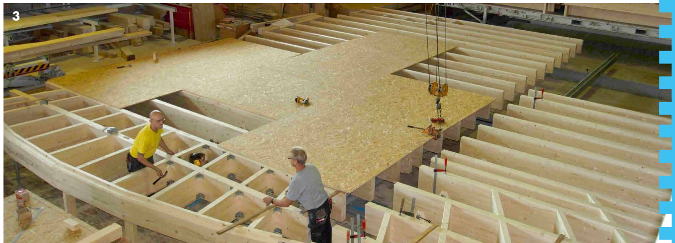
3 / Restaurant: 40 cm hohe Geschosdecke mit gekrümmtem Radträger und ausgespartem Unterzug auf tectofix 3000
