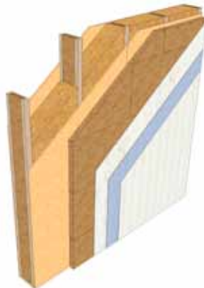
WDVS auf Holzrahmenkonstruktion mit Plattenwerkstoff
